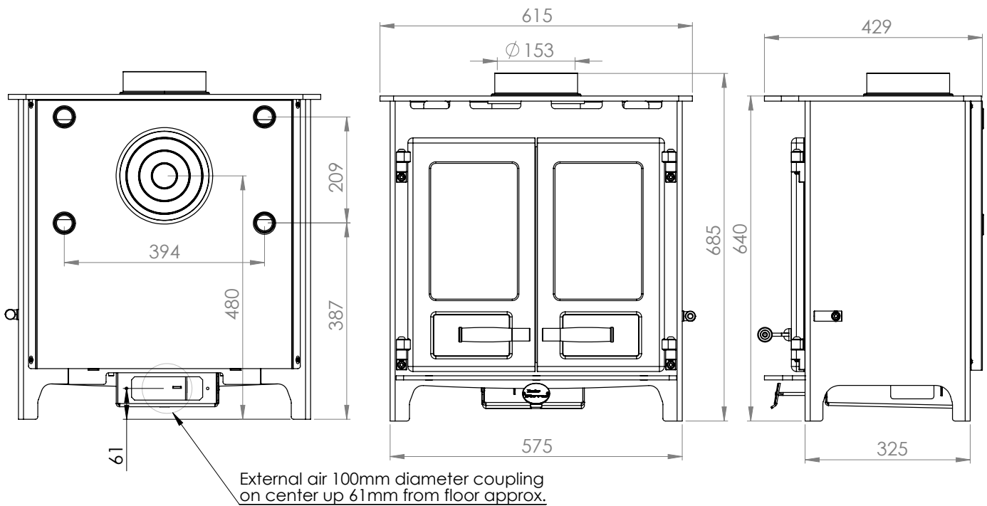
InisOirr MK 2 BOILER
