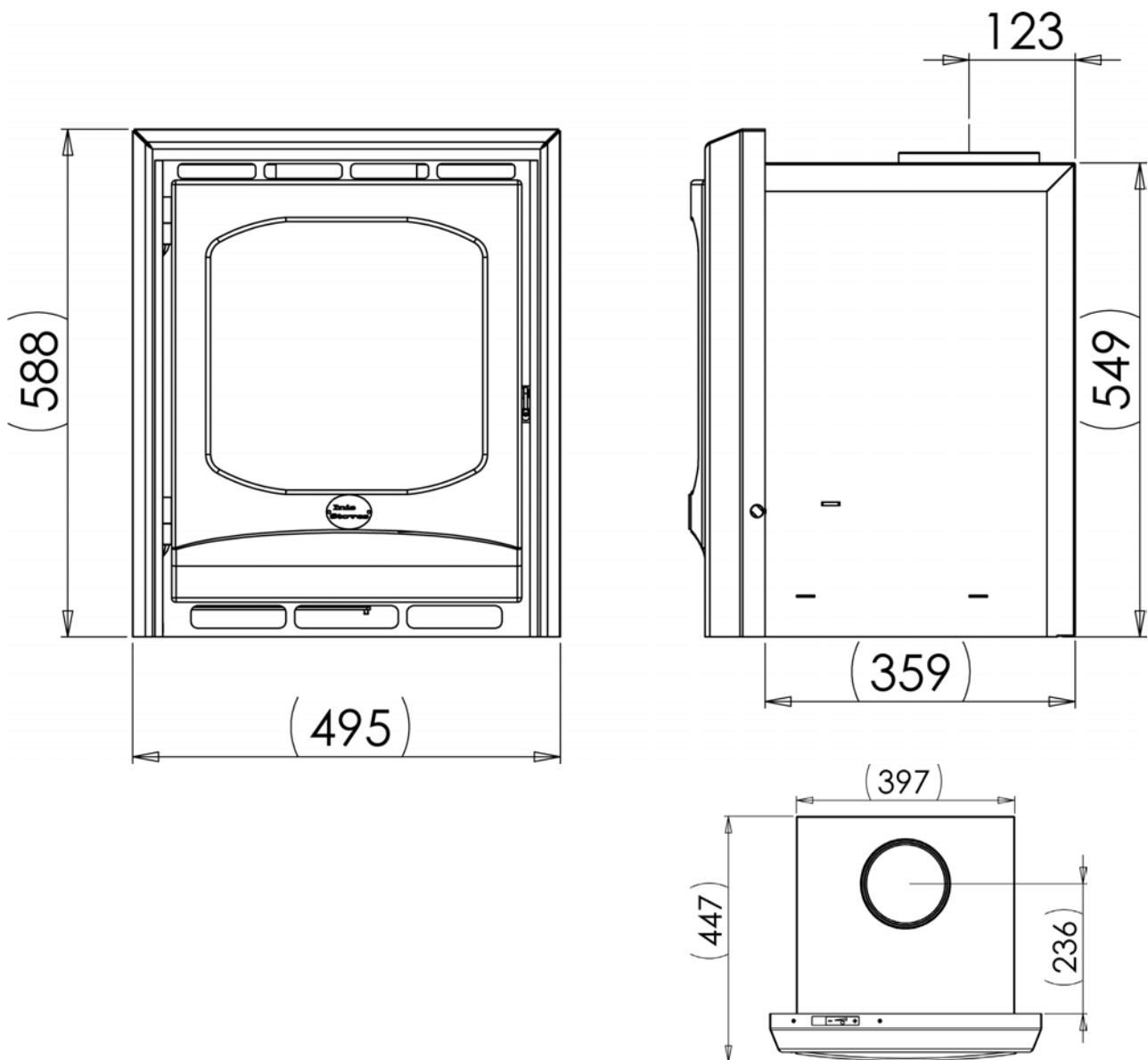
InisBofin INSERT STOVES
