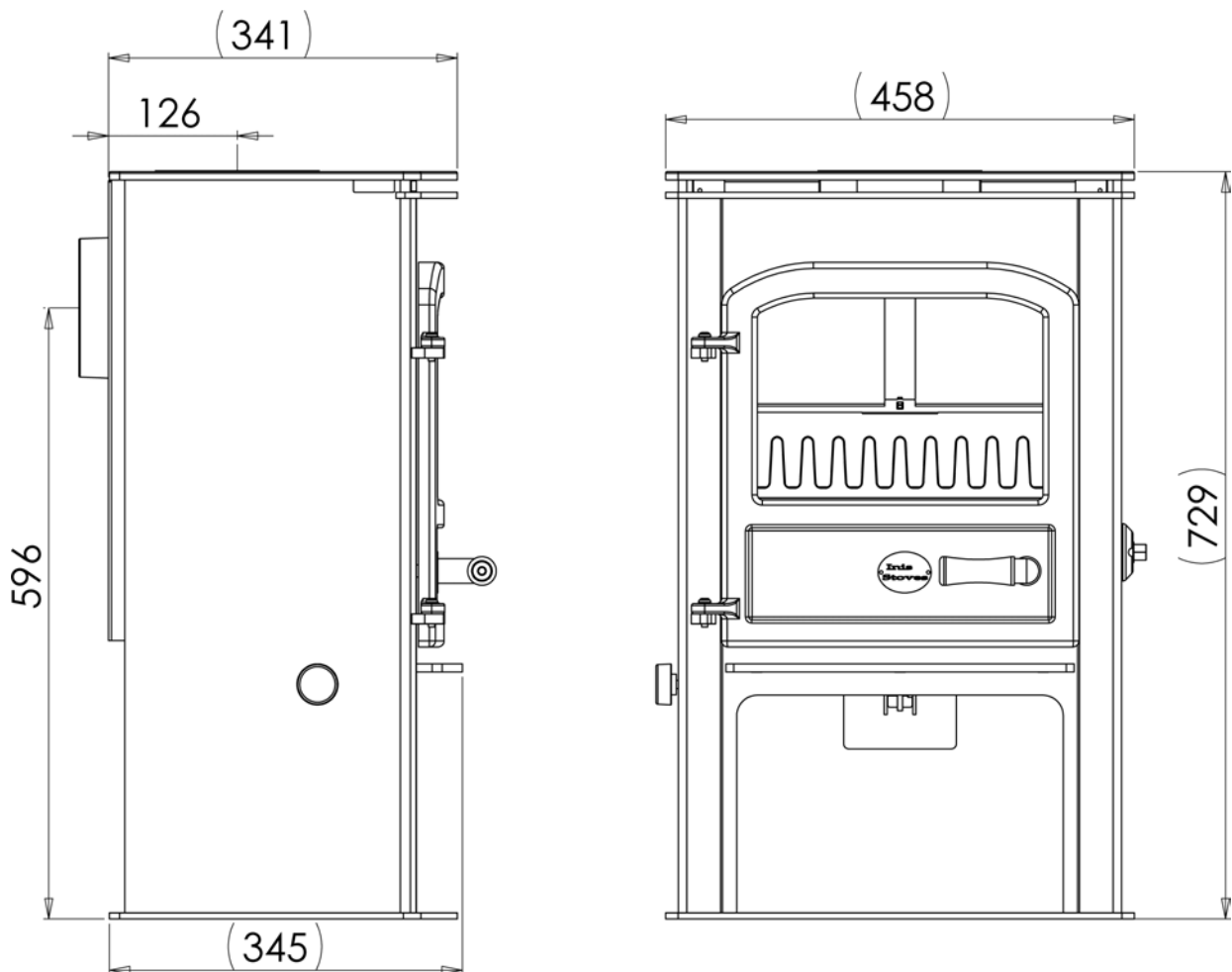
InisAirc Ard ROOMHEATER
