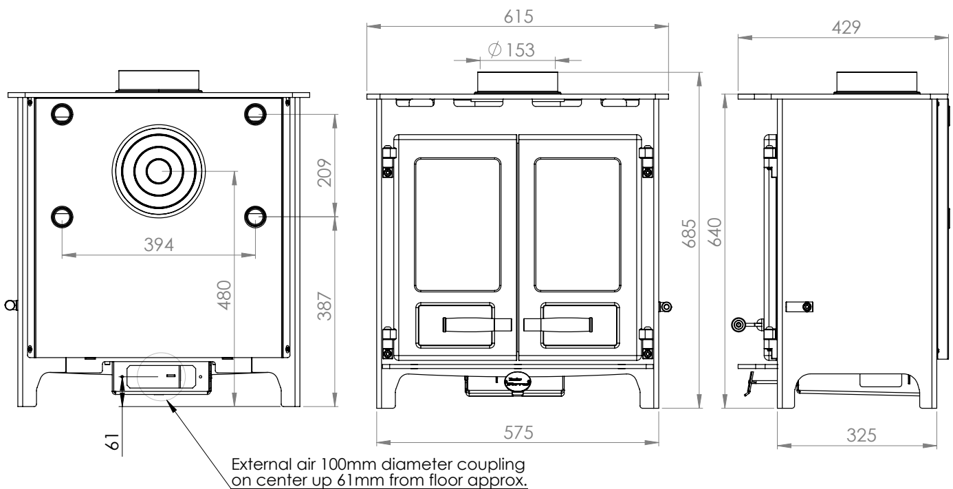
InisOirr MK 2 ROOMHEATER
